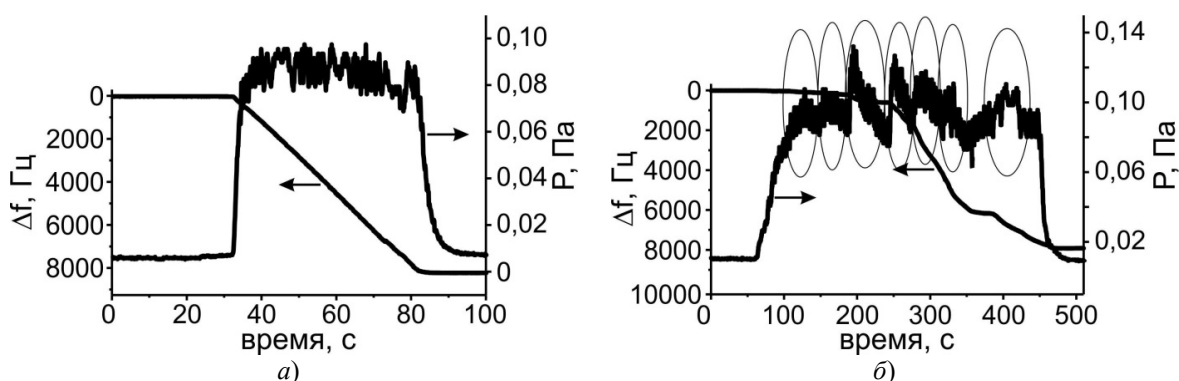
Рисунок 2.1 – Кинетика электронно-лучевого диспергирования ПТФЭ (а) и смеси \text{Fe}(\text{NO}_3)_3 \cdot 9\text{H}_2\text{O} + \text{Al} + \text{ПТФЭ} (б)
