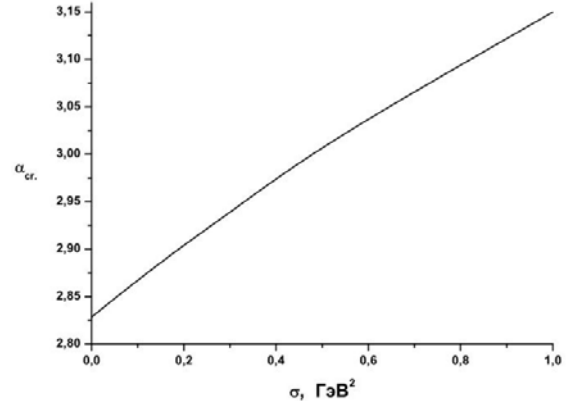
Рисунок 1 – Зависимость критического значения \alpha_{crit} от параметра линейного запирающего \sigma для уравнения Шредингера
